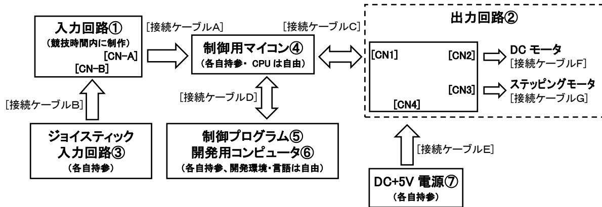
図1 課題システムの構成
